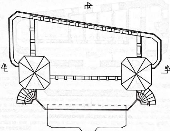
PIANTA DELLE COPERTURE
